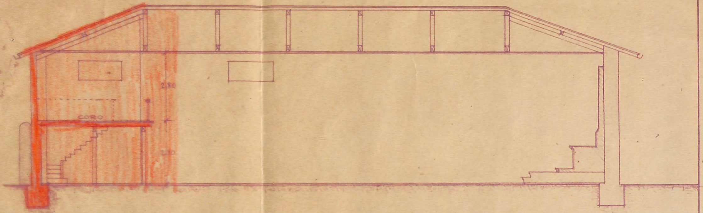
SECCIÓN LONGITUDINAL
