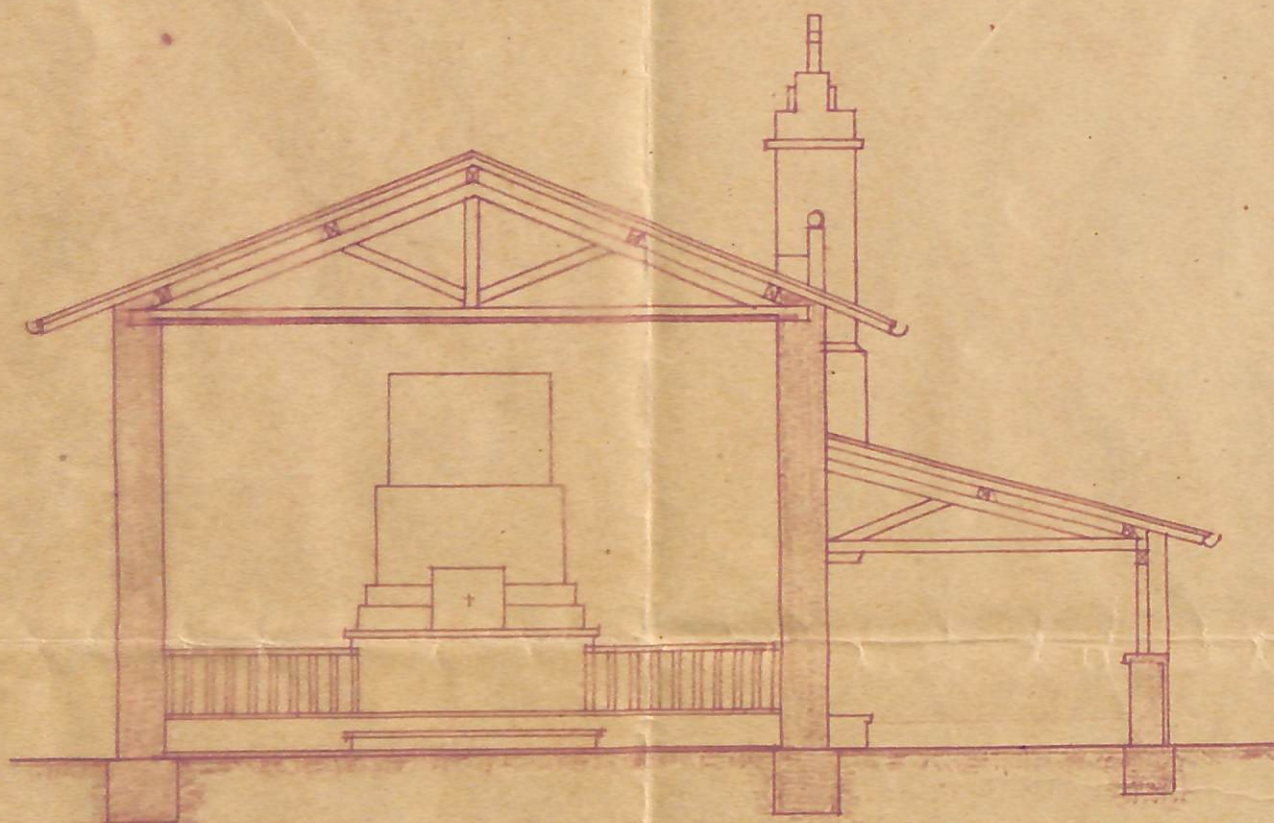
SECCIÓN TRANSVERSAL
